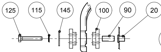
ESPLOSO FISSAGGIO BRACCI MRE A FCT
