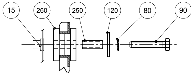
ESPLOSO FISSAGGIO BRACCI MRE A FCT
